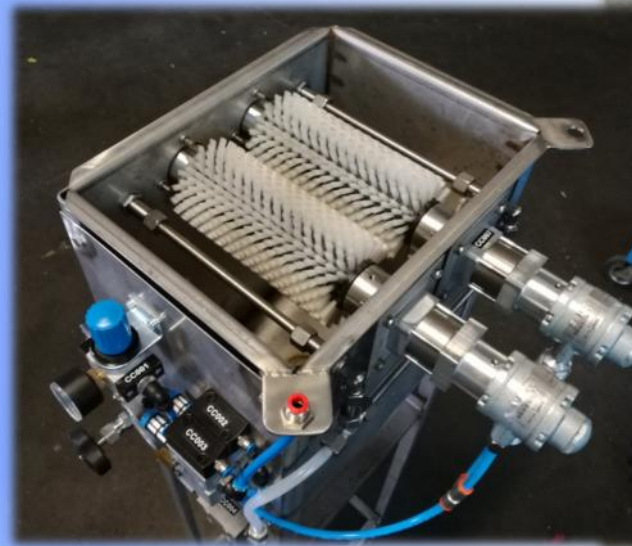
Dispositivi di pulizia CAP CLEANER per apparecchiature automatiche e coppe
