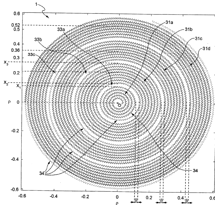
Figura 2 – Distribuzione delle aperture sulla superficie dell'antenna
