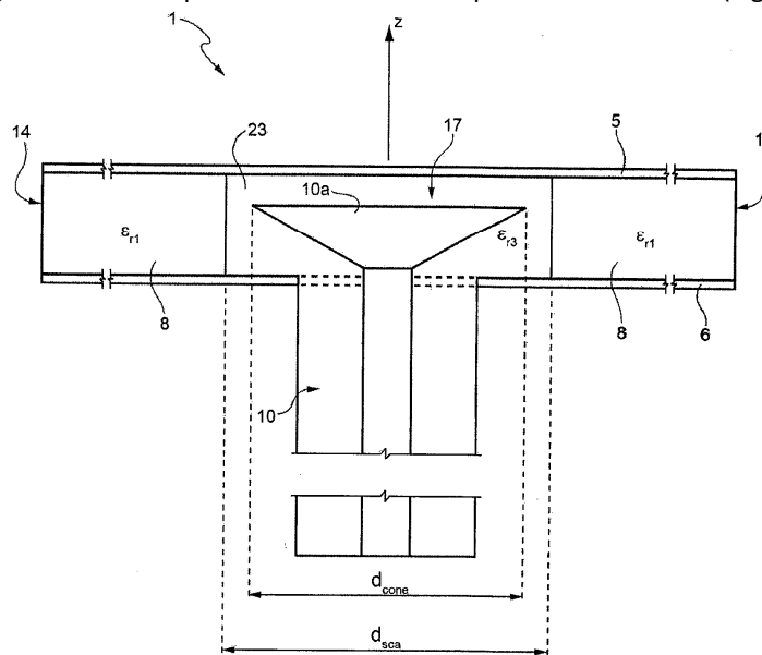
Figura 1 – Struttura dell'antenna a guida d'onda
